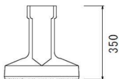
B 型（根石、天端型）
