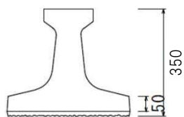
A 型（標準型）
