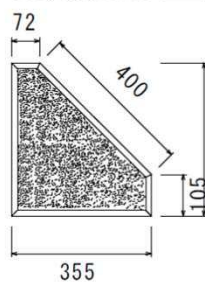
E 型（隅角型）
